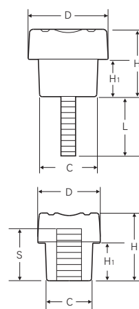
寸法図
