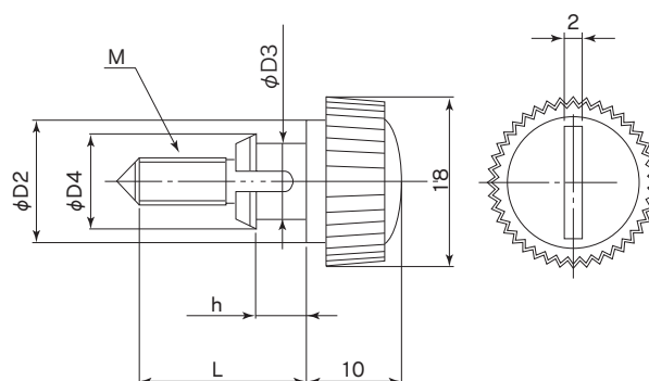
寸法図
