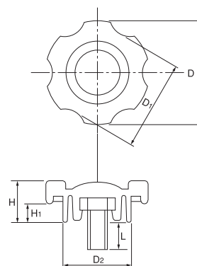
寸法図
