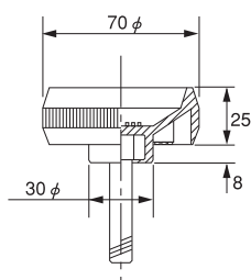
寸法図
