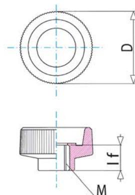
ナット
