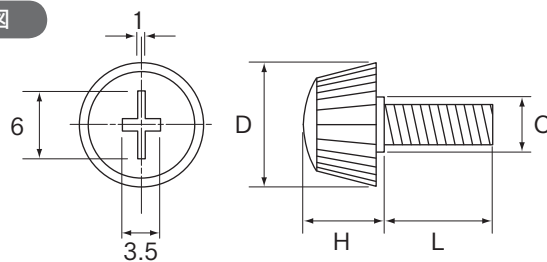
●寸法表 (m/m)
