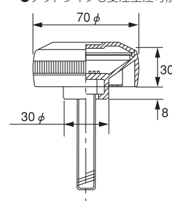
寸法図
