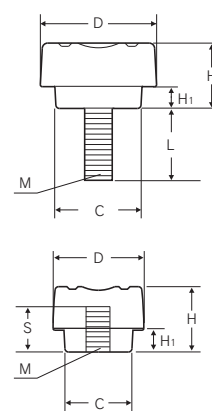
寸法図
