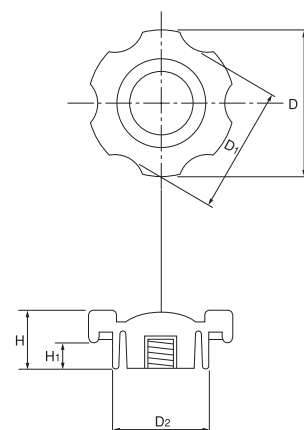
寸法図
